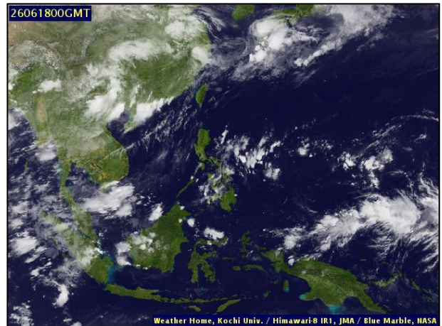
ภาพถ่ายดาวเทียม วันที่ ๑๘ มิ.ย. ๒๕๖๙ เวลา ๐๗.๐๐ น.
